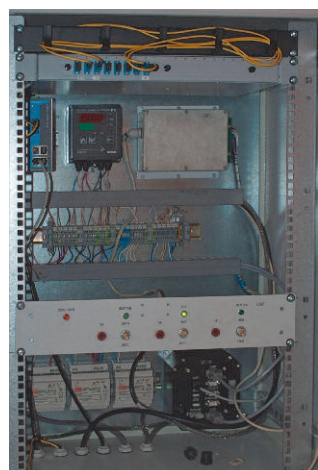
Рис. 4. Шкаф контроллера управления и дополнительных устройств
